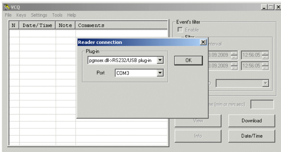
Рис. 2: Подменю Connection
